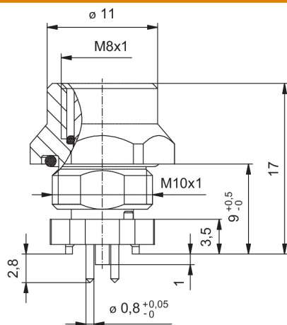
Габаритный чертёж
