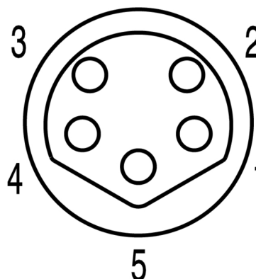
Схема контактов
