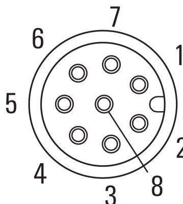
Схема контактов
