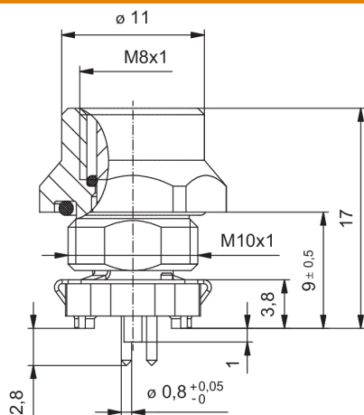
Габаритный чертёж
