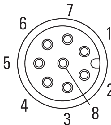
Схема контактов
