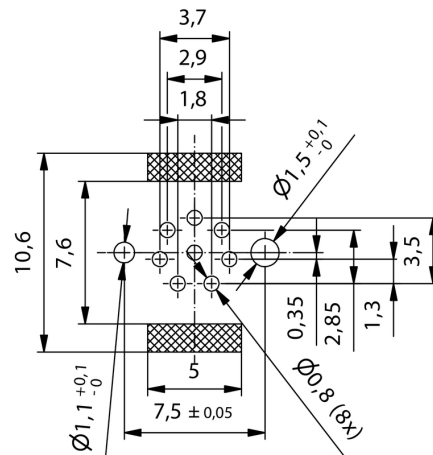
Чертеж PCB платы
