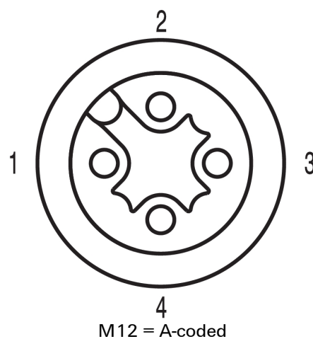
Schemat biegunów
