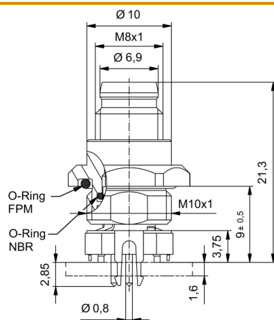
Габаритный чертеж
