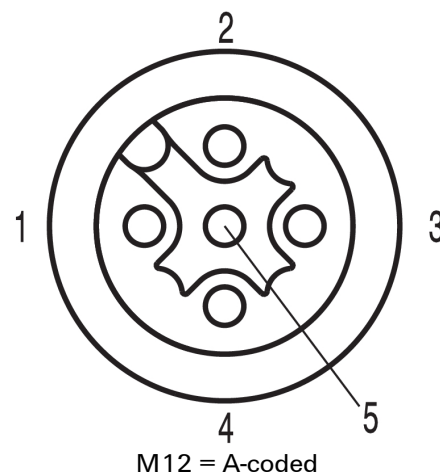
Схема контактов
