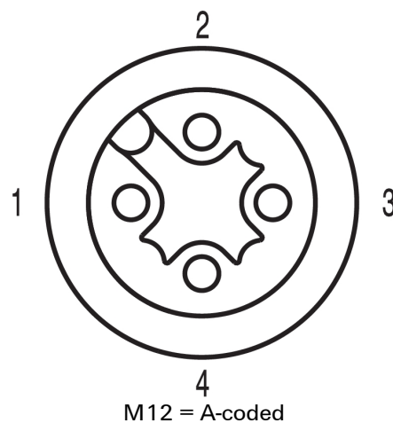
Схема контактов
