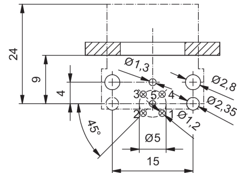
Schemat biegunów
