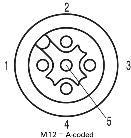
Schemat biegunów
