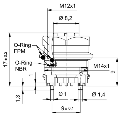
Габаритный чертёж
