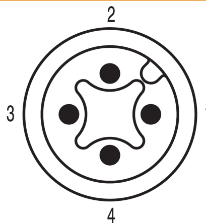
Schemat biegunów
