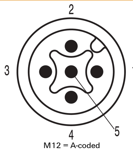
Схема контактов
