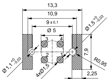
Чертёж РСВ платы
