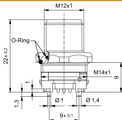
Габаритный чертёж
