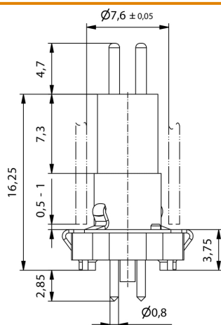
Габаритный чертеж
