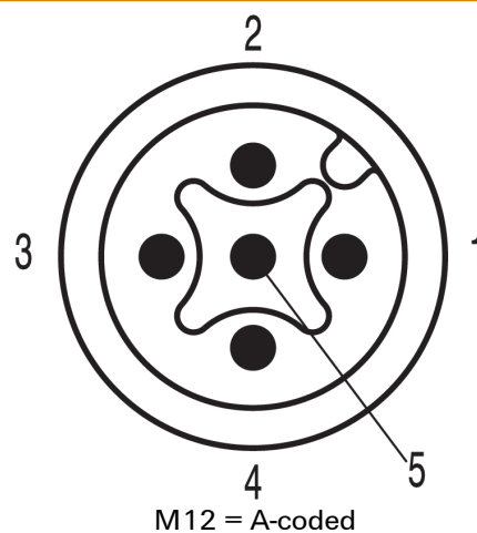
Схема контактов
