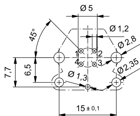
Чертеж PCB платы
