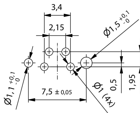
Чертеж PCB платы
