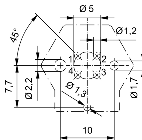
Чертеж РСВ платы
