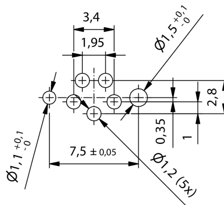
Чертеж PCB платы
