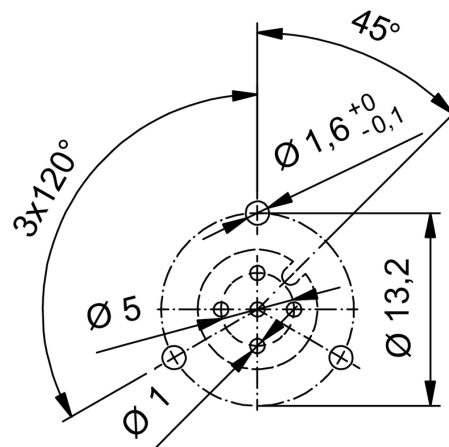
Схема контактов
