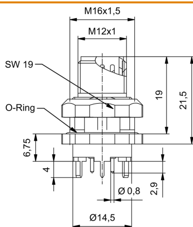
Rysunek wymiarowy
