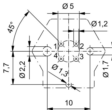
Схема контактов
