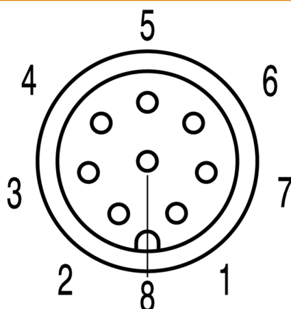
Схема контактов
