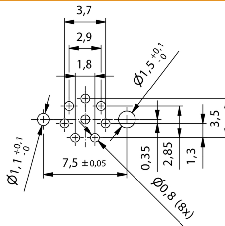
Чертеж РСВ платы
