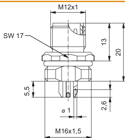
Габаритный чертеж
