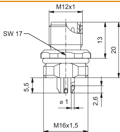
Rysunek wymiarowy
