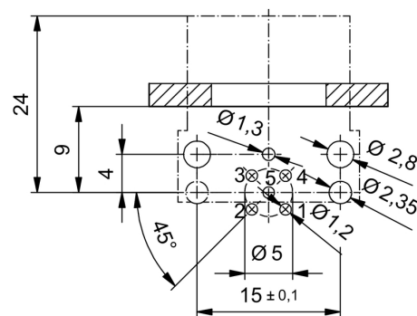
Схема контактов
