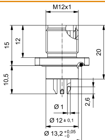
Габаритный чертеж
