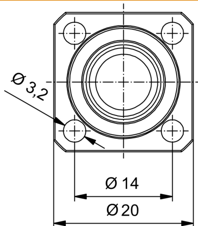
Wycięcie montażowe
