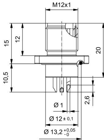
Rysunek wymiarowy
