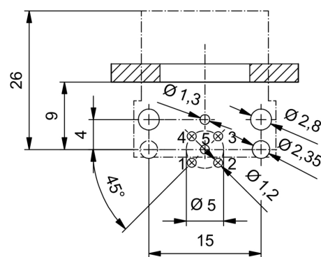
Чертеж PCB платы
