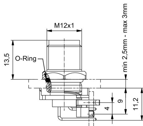
Габаритный чертеж
