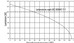
HP 200 / IP65-Gehäuse / 4 Pole
