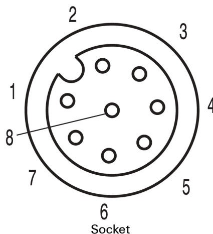
Socket
