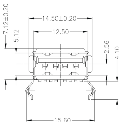
Rysunek wymiarowy
