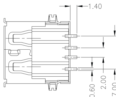
Rysunek wymiarowy
