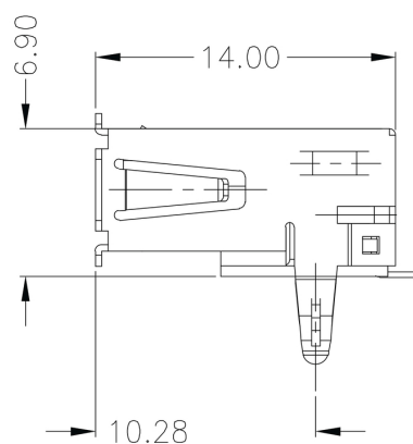
Rysunek wymiarowy
