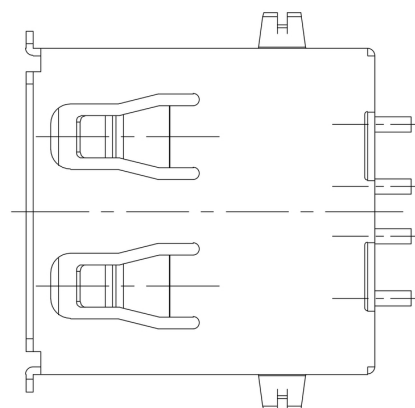
Rysunek wymiarowy
