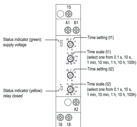
Детальный чертеж
