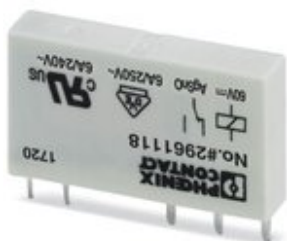
Steckbares Miniaturleistungsrelais, mit Leistungskontakt, 1 Wechsler, Eingangsspannung 60 V DC
