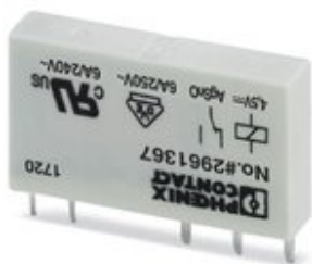
Steckbares Miniaturleistungsrelais, mit Leistungskontakt, 1 Wechsler, Eingangsspannung 4,5 V DC
