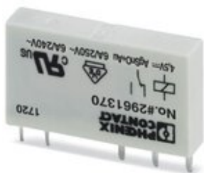
Steckbares Miniaturleistungsrelais, mit Mehrlagen-Goldkontakt, 1 Wechsler, Eingangsspannung 4,5 V DC
