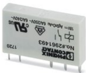
Steckbares Miniaturleistungsrelais, mit Mehrlagen-Goldkontakt, 1 Wechsler, Eingangsspannung 18 V DC
