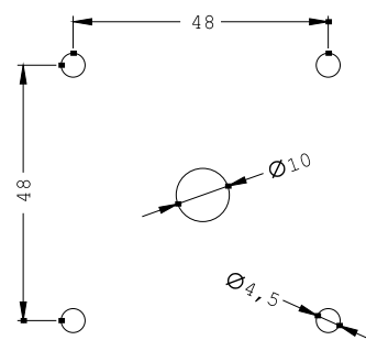
Bohrbild Tuer
