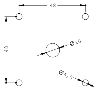
Bohrbild Tuer
