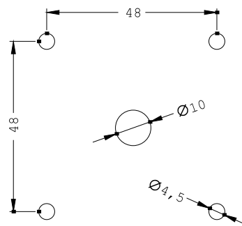
Bohrbild Tuer
