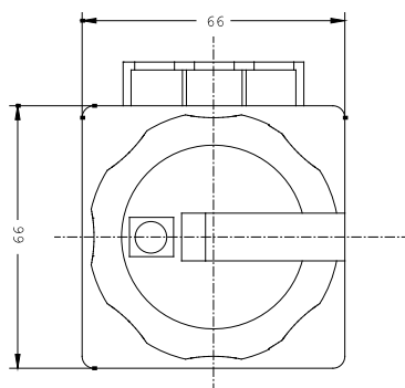
Bohrbild Tuer
