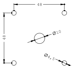
Bohrbild Tuer
