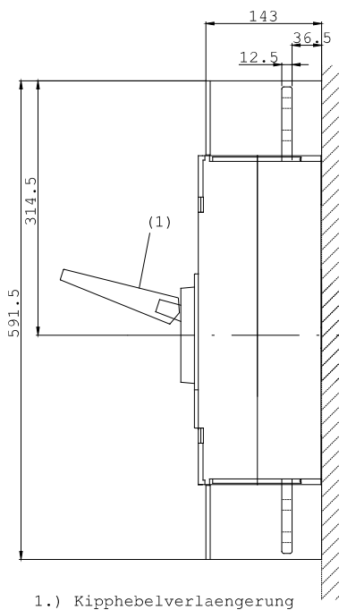
1.) Kipphebelverlaengerung
