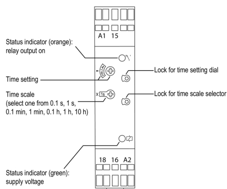
Детальный чертеж
