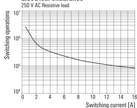
Trwałość elementów elektrycznych 250 V AC obciążenie rezystancyjne
