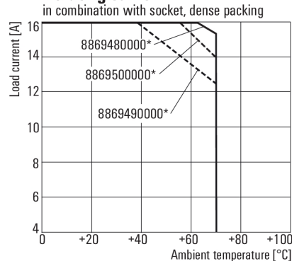
Krzywa obciążalności prądowej Przełącznik połączony z podstawką
