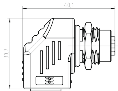
Габаритный чертеж
