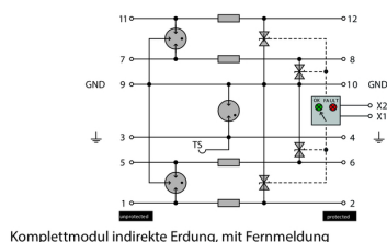
Komplettmodul indirekte Erdung, mit Fernmeldung Komplettmodul
