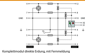
Komplettmodul direkte Erdung, mit Fernmeldung
