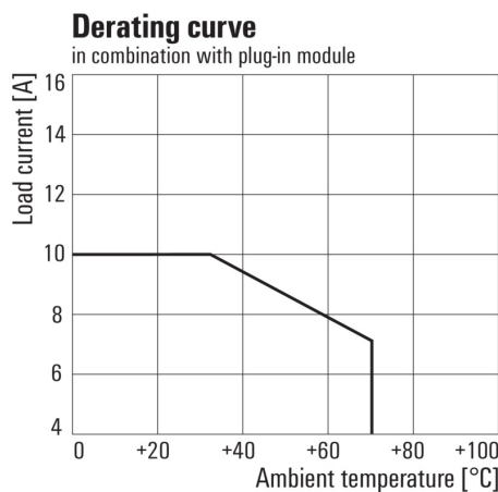
Deratingcurve Relais in Kombination mit Sockel
